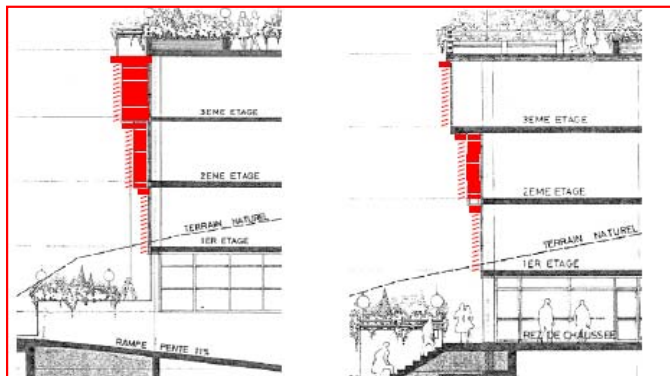
Figure 2 : Intégration d'un système de store extérieur (vues en coupe)
